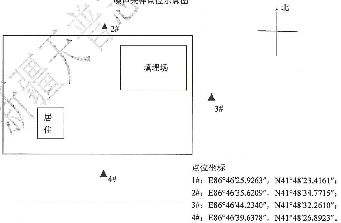
噪声采样点位示意图
